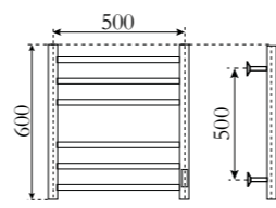
Высота 600 мм вставки: 3+3
