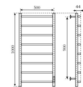
Высота 1000 мм вставки: 8
