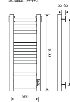
Высота 100 Вставки: 3+4+3
