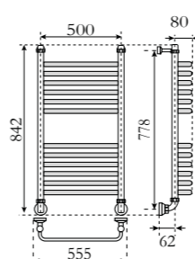
Высота 800 мм вставки: 6+6
