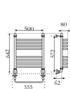
Высота 600 мм вставки: 4+4
