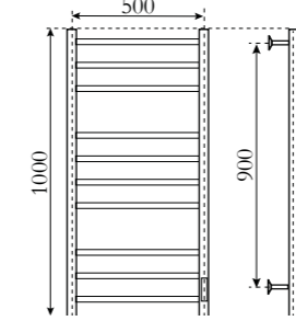
Высота 1000 мм вставки: 3+4+3
