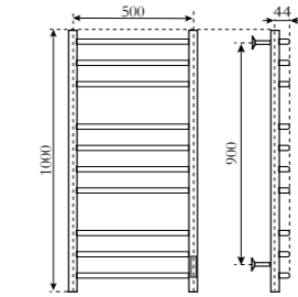
Высота 1000 мм вставки: 8
