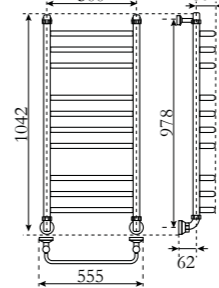
Высота 1000 мм вставки: 3+5+7
