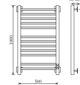
Высота 100 Вставки: 5+5+2
