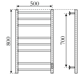
Высота 800 мм вставки: 3+3+2
