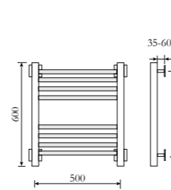
Высота 60 Вставки: 4+4
