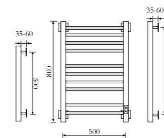
Высота 80 Вставки: 4+4+2
