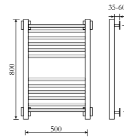
Высота 80 Вставки: 6+6
